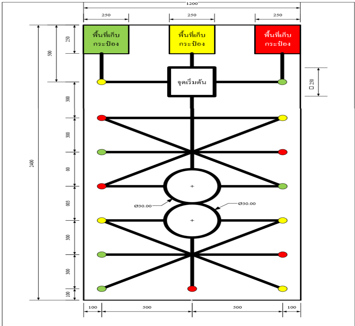
ภาพจำลองสนามหุ่นยนต์อัตโนมัติระดับมัธยมศึกษาปีที่ ๔ - ๖
