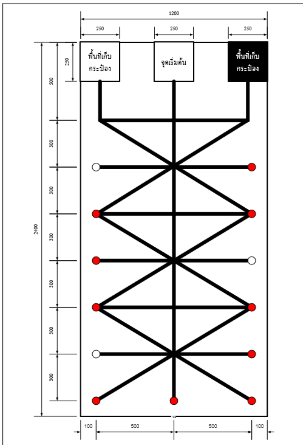
ภาพจำลองสนามแข่งขันหุ่นยนต์อัตโนมัติ ระดับมัธยมศึกษาปีที่ ๑ - ๓
